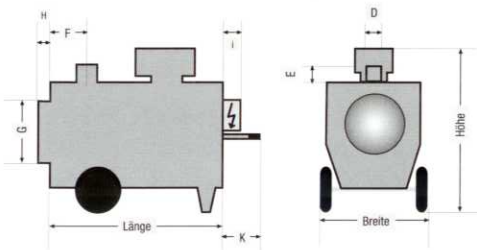
Typenreihe K · Maße in mm
